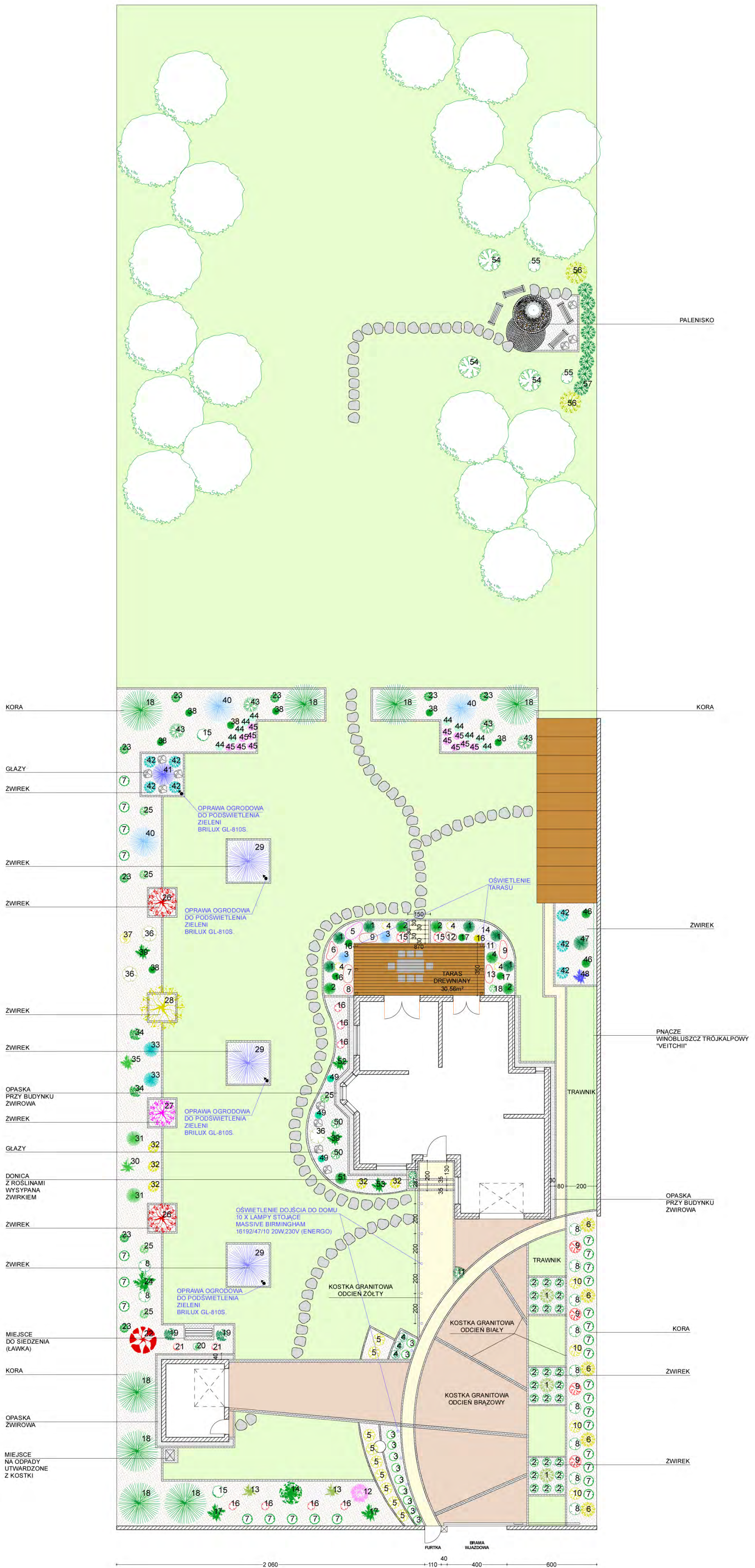
PROJEKT OGRODU RZUT SKALA 1:150
