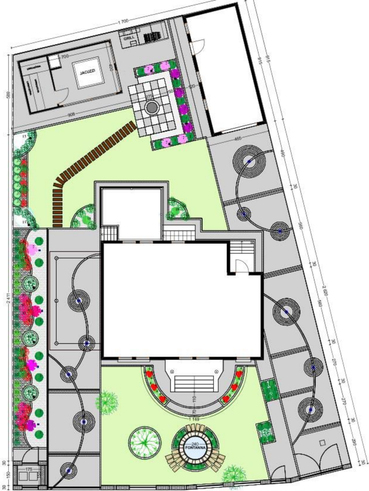
PROJEKT ZAGOSPODAROWANIA OGRODU RZUT SKALA 1:50
